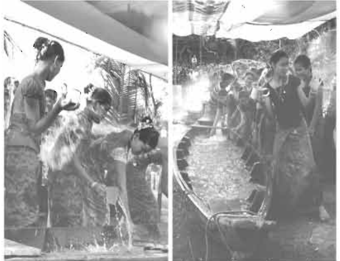
চিত্র- ৬.৩ : মারমা ও রাখাইন নৃগোষ্ঠীর পানিখেলা উৎসব
