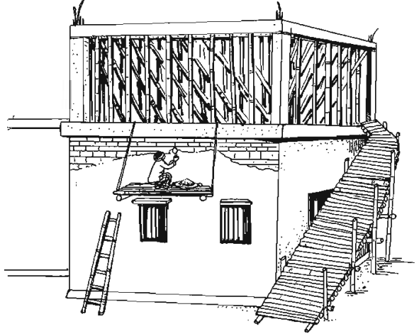
চিত্র : দালানকোঠা নির্মাণে বাঁশ
